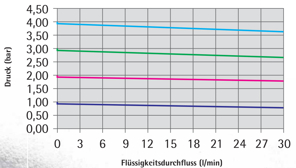
Durchflusskurve mit CO 2
