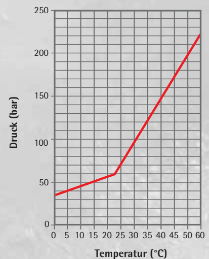
Füllverhältnis 0,746 kg/l
